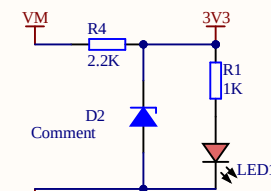
电源指示灯
