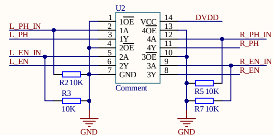
缓冲电路
