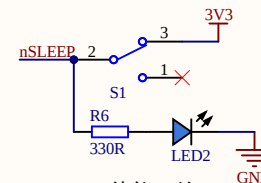
使能开关
